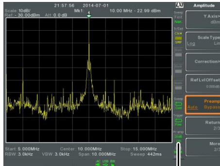
Pr-amp icon
