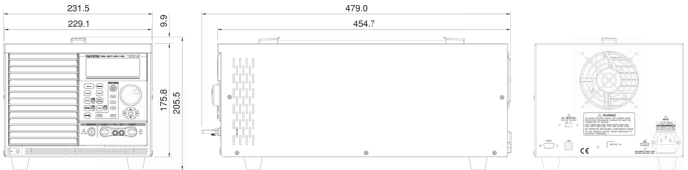
PEL-507-80-140 / PEL-507-500-30
